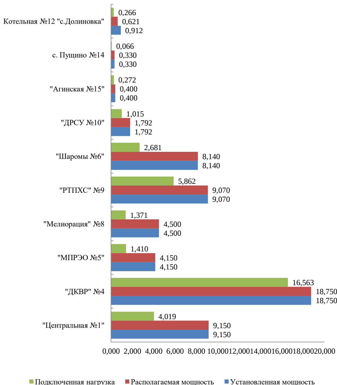
Рис. 2.1.5 – Распределение мощностей источника тепловой энергии
