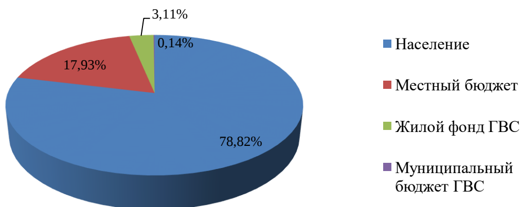
Рис.1.2 – Потребление тепловой энергии на отопление и ГВС по потребителям от котельной №4 «ДКВР»
