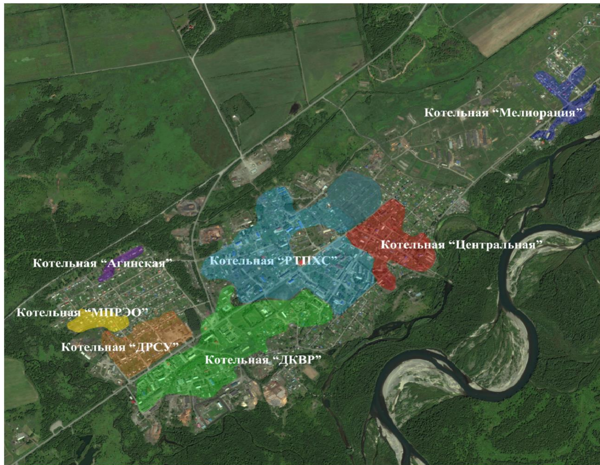
Рис. 2.1.1 – Зона действия системы теплоснабжения села Мильково
