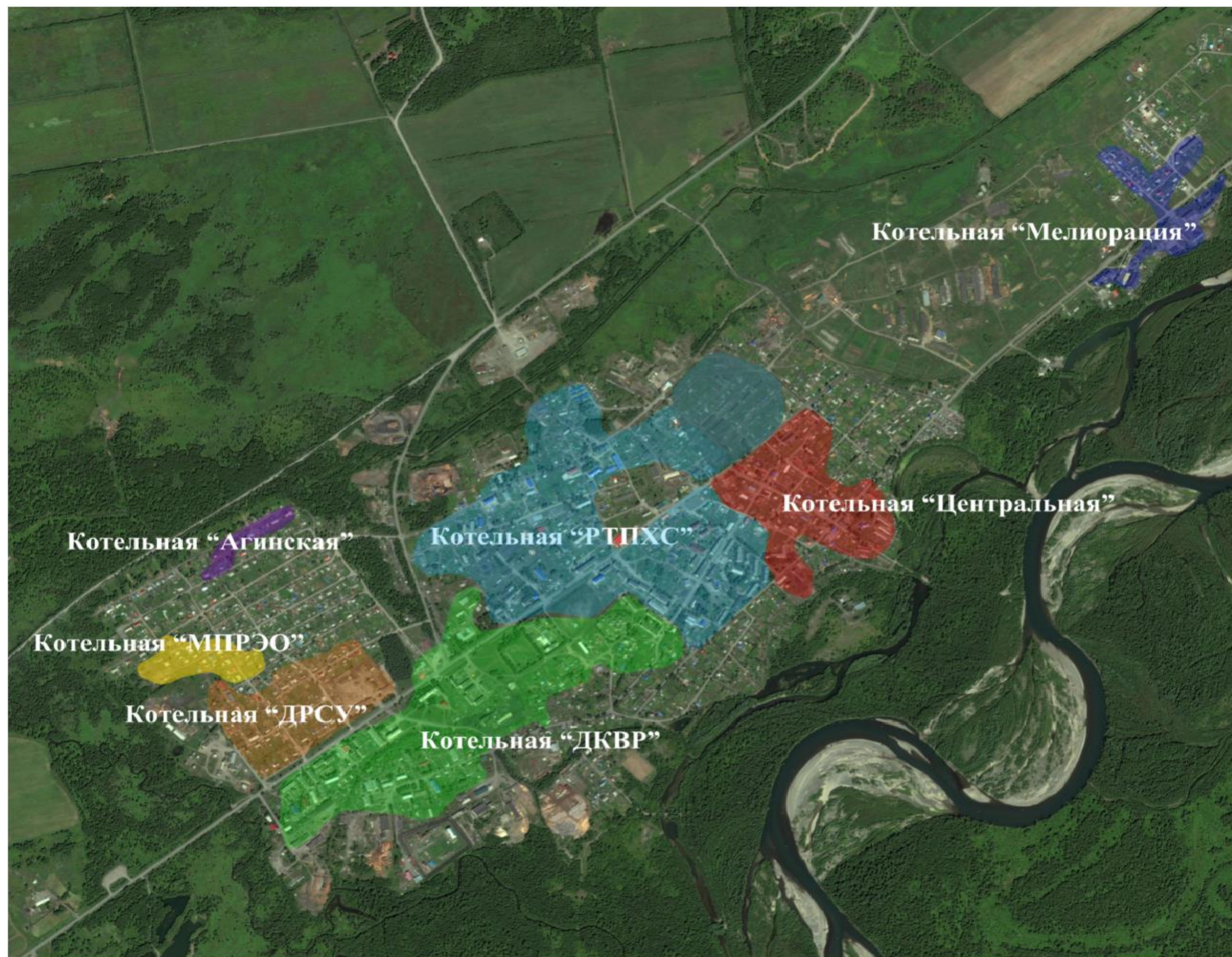
Рис. 1.2.1 – Зона действия системы теплоснабжения села Мильково
