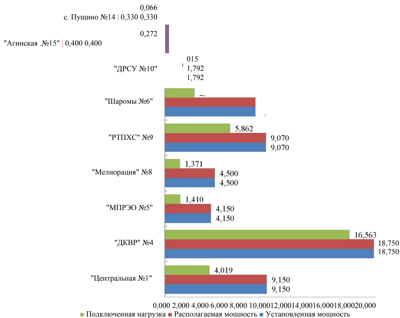
Рис. 2.1.5 - Распределение мощностей источника тепловой энергии
