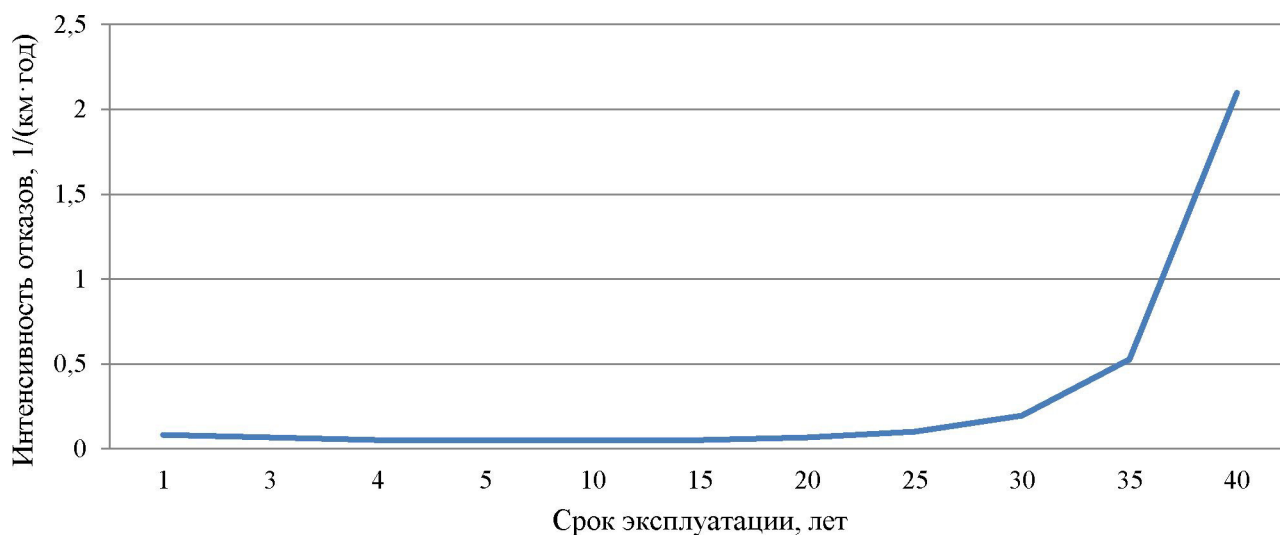
Рис. 2.1.7 - Интенсивность отказов в зависимости от срока эксплуатации участка тепловой сети
