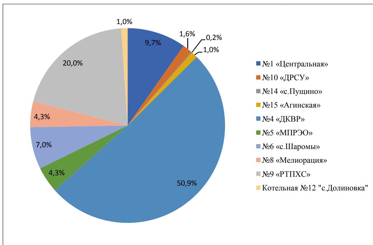
Рис. 1.7 - Удельный вес источников теплоснабжения по выработке тепловой энергии муниципального образования «Мильковское сельское поселение»
