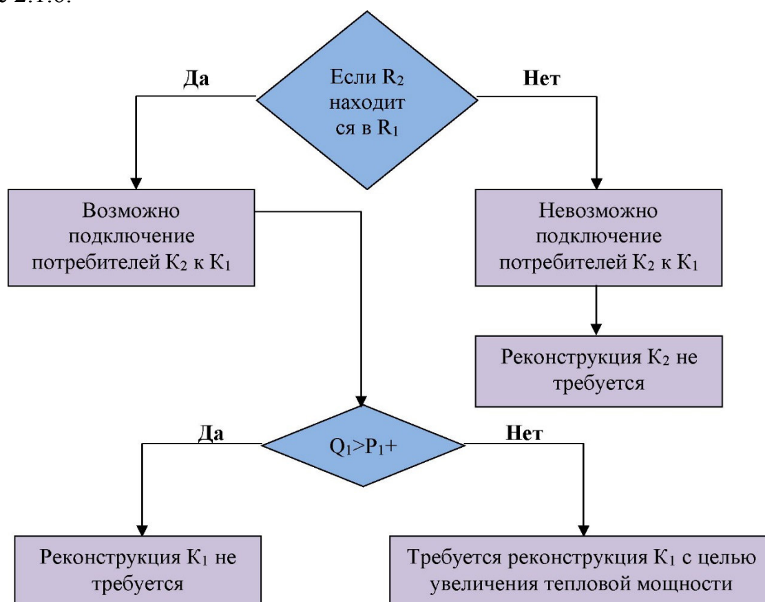
Рисунок 2.1.6 - Блок-схема обоснования реконструкции котельной
